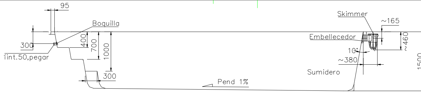
SECCION A-A'
