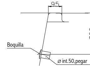
DETALLE B
