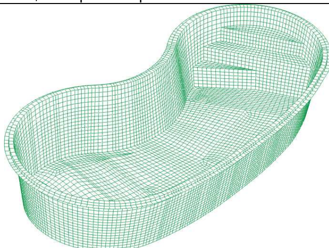
Mallado de nodos para análisis de Resistencia de Materiales por Elementos finitos
