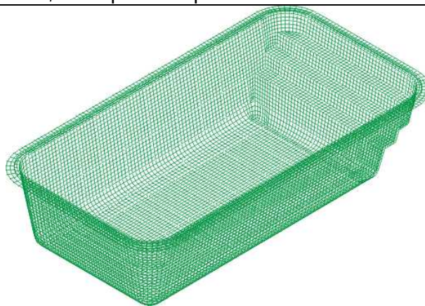
Mallado de nodos para análisis de Resistencia de Materiales por Elementos finitos
